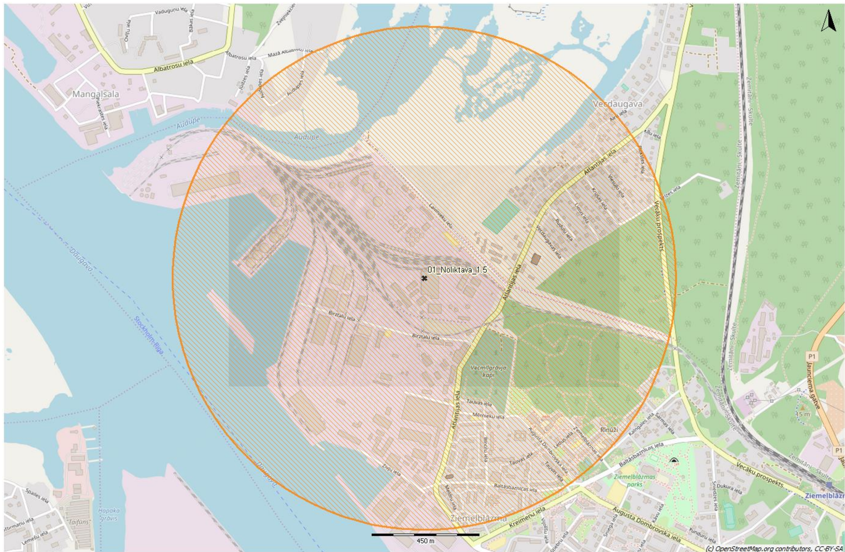
1.3. attēls. Maksimālās 1% letālās iedarbības distance ugunsgrēka gadījumā, kā rezultātā notiek kālija nitrāta termiska sadalīšanās ķīmisko vielu uzglabāšanas noliktavā
